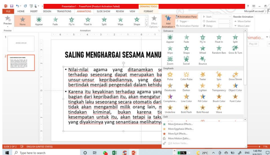
Gambar 3. Penambahan Animasi
