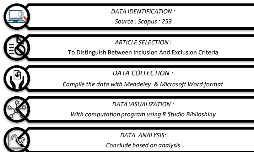
Gambar 1. Desain Pencarian
